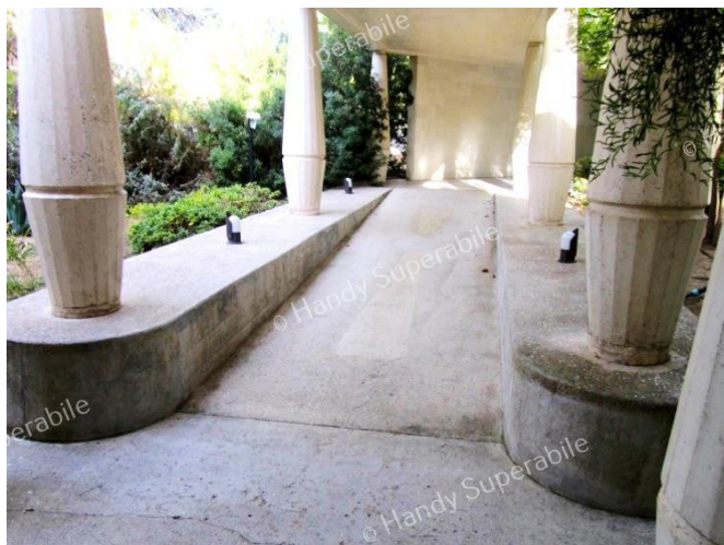
La rampa di accesso al ristorante con pendenza del 7%
